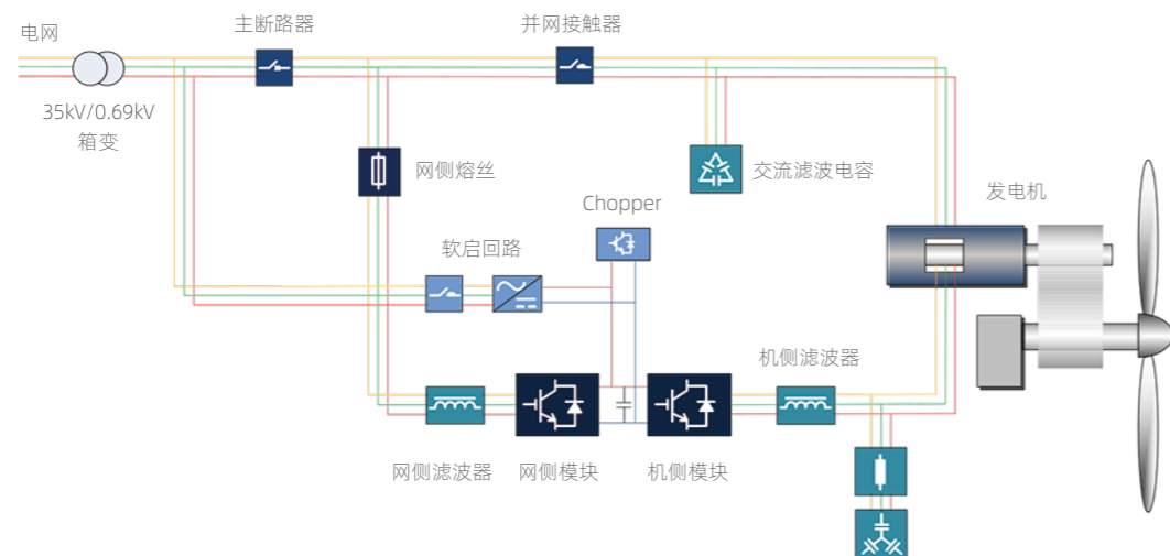
690V双馈风力发电系统结构图
